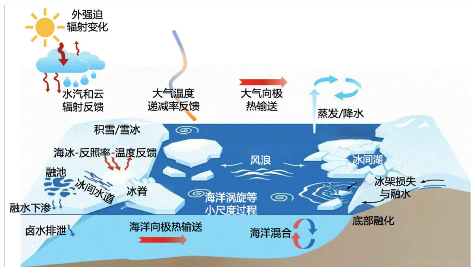
图 6 极地快速变化的关键过程
