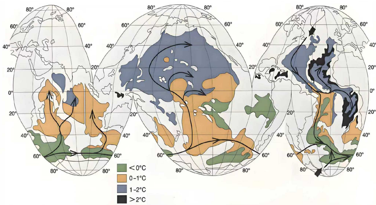
图7 深海环流 [47]
