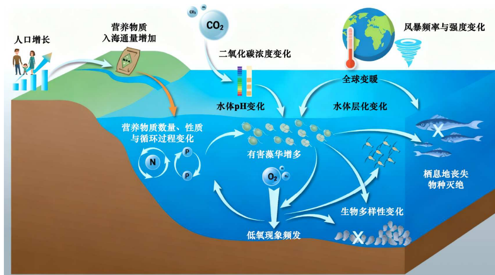
图 9 复合胁迫作用下河口-近海系统的韧性调控 [60]
