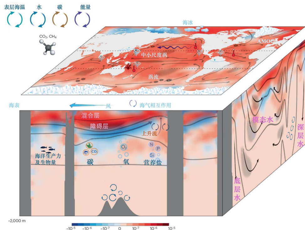
图 10 海洋动力过程对碳-氮-氧生物地球化学循环的影响 [68]
