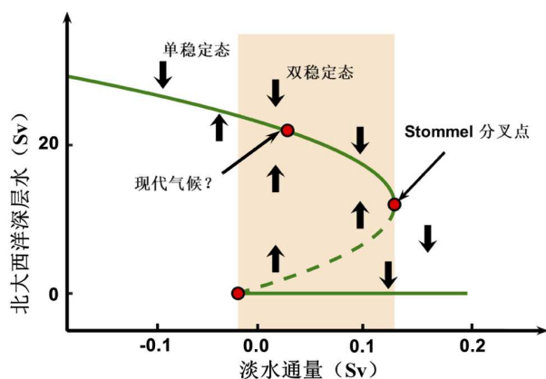
图8 大洋热盐环流变化的临界点 [51]
